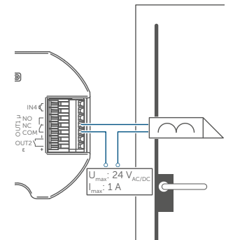
B: Elektryczny otwieracz drzwi z funkcją zamkniętego obwodu
