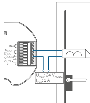
A: Klasyczny elektryczny otwieracz drzwi
